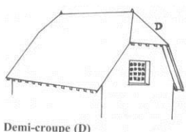
avec une demi-croupe
