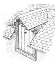
lucarne pendante, dite meunière, ou à foin
